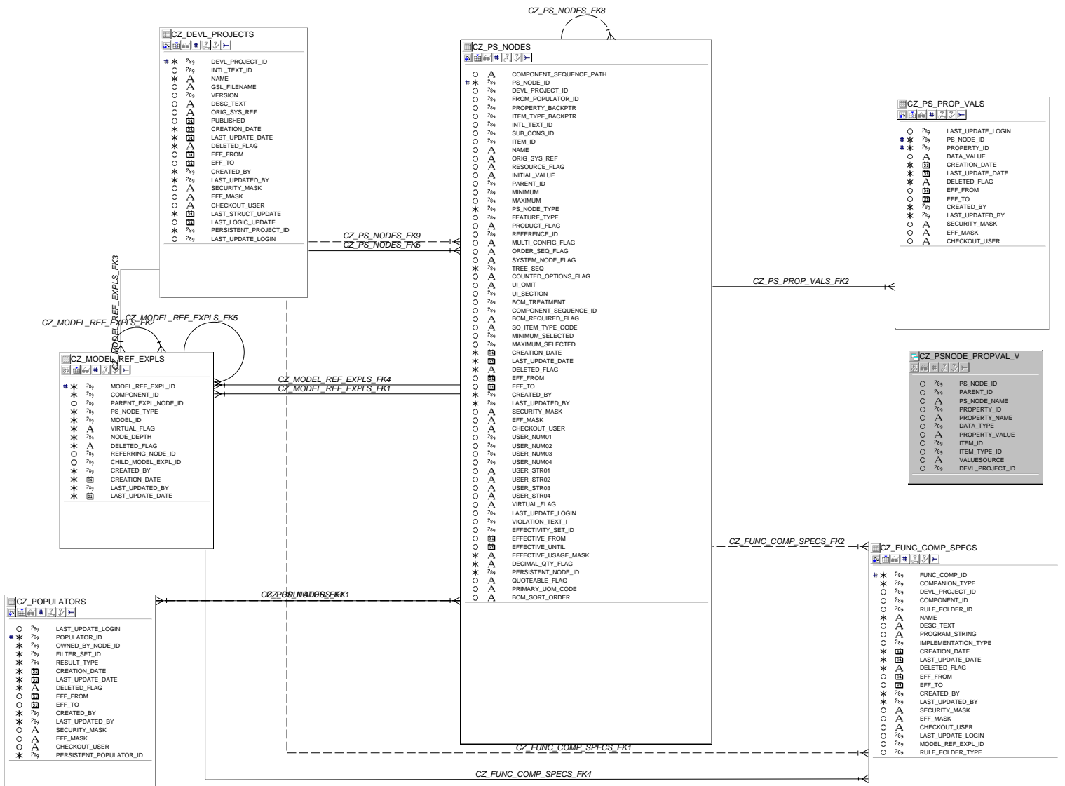
Diagram : CZ_115_F_16D_PROJ Title : PROJ - Configurator Project Structure
